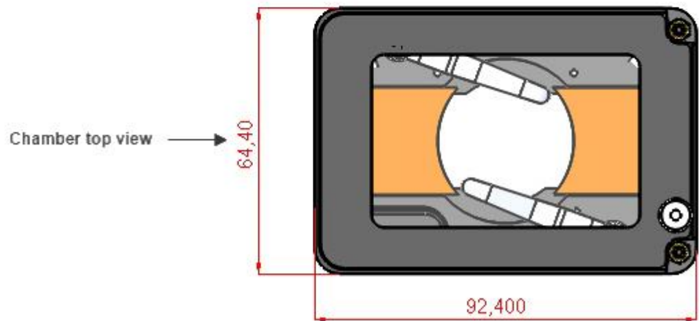
H201-PI-P-736-ZR1S/ZR2S - Dimensions
